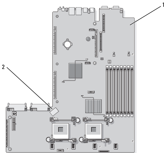
1 システム基板 2 内部 USB コネクタの位置
